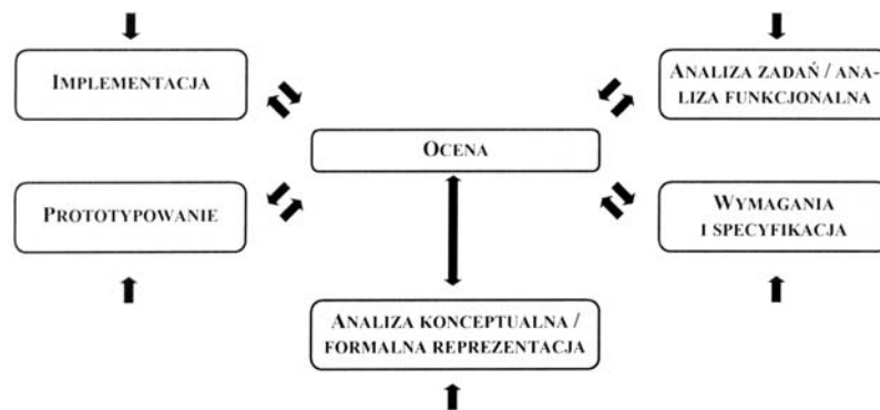
Rys. 5. Model gwiazdy cyklu życia oprogramowania Źródło: Opracowanie własne na podstawie prac: [18], [33].
